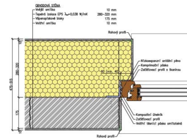
Obr. 13 Detail musí obsahovat kromě izolace i způsob těsnění včetně vnitřního a vnějšího uzávěru. Pro připojení parapetu i okna se z vnější strany používají komprimační pásy, které chrání spáru před vnikem hnaného deště.
