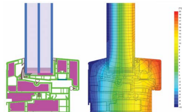
Obr. 5 Optimalizované dutiny a řešení těsnících rovin zvyšuje teploty ve funkční spáře a zabráňuje tvorbě kondenzátu a namrznání. Perfektní řešení geometrie parapetu plastových oken nové generace. (Zdroj FBS OVER VADB 550+)
