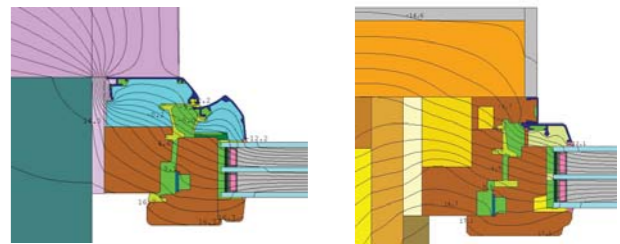
Obr. 10 Výřez z 2D simulace dřevohliníkového okna (vlevo). Vnější přezizolování rámu pozbývá svou funkci, protože vysoce vodivý hliníkový profil posouvá izotermu hluboko dovnitř izolace. Naproti tomu optimalizovaný dřevohliníkový profil obsahuje jen malou hliníkovou lištu a celý rám je spolehlivě ochráněn vnější izolací. 2D simulace jsou výbornou pomůckou při optimalizaci osazení oken.
