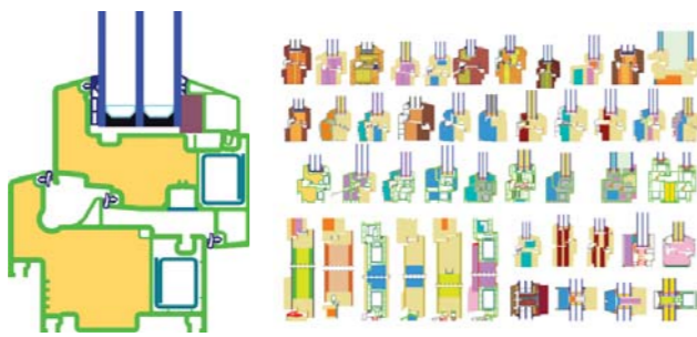
Obr. 3 Řez oknem pro pasivní domy. Na trhu je dnes dostupná řada ráků certifikovaných v Passivhaus Institutu v Německu. (Zdroj PHI)
