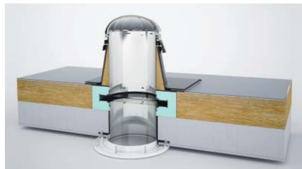
Obr. 11 Tepelně vhodnější variantou je světlovod. Výrobci již reagují na požadavky pasivních domů speciální tvarovkou s vloženým trojsklem. Výsledkem je ideální osazení v konstrukci izolace. (Zdroj Lightway)
